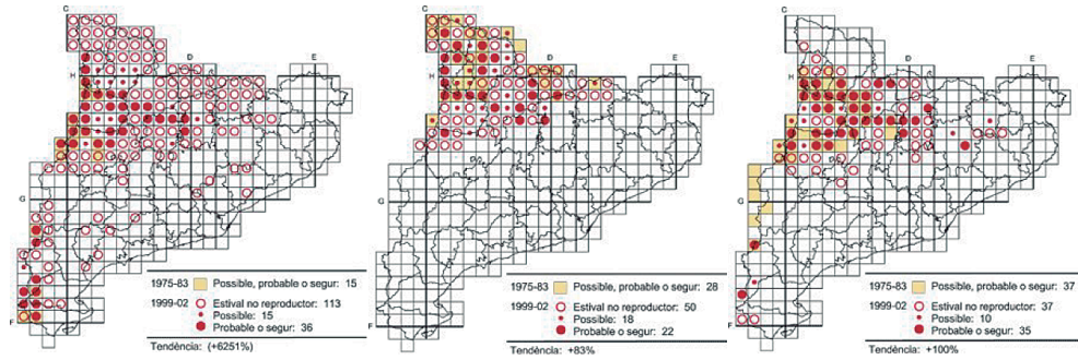
FIGURA 2. Mapes de distribució de la zona de nidificació del voltor comú, del trencalòs i de l'aufrany (Estrada et al. , 2004).
